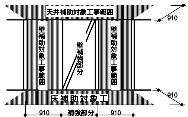
【例1】 耐力壁(筋交い)を設置した場合
