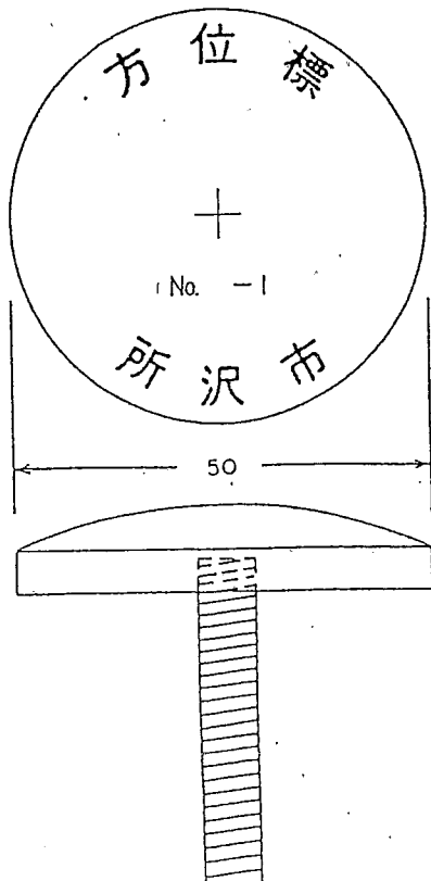
方位標金属標及び埋標構造図
