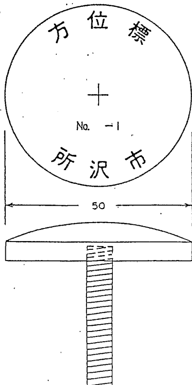
方位標金属標及び埋標構造図
