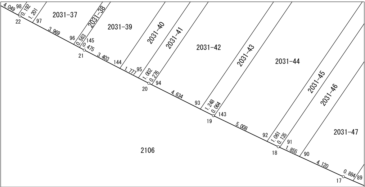
S=1/200
