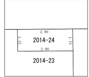
拡大図D S=1 : 100
