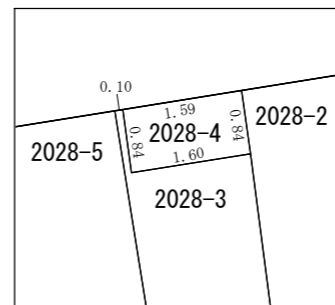
拡大図A S=1 : 100
