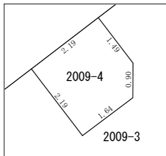
拡大図B S=1 : 100
