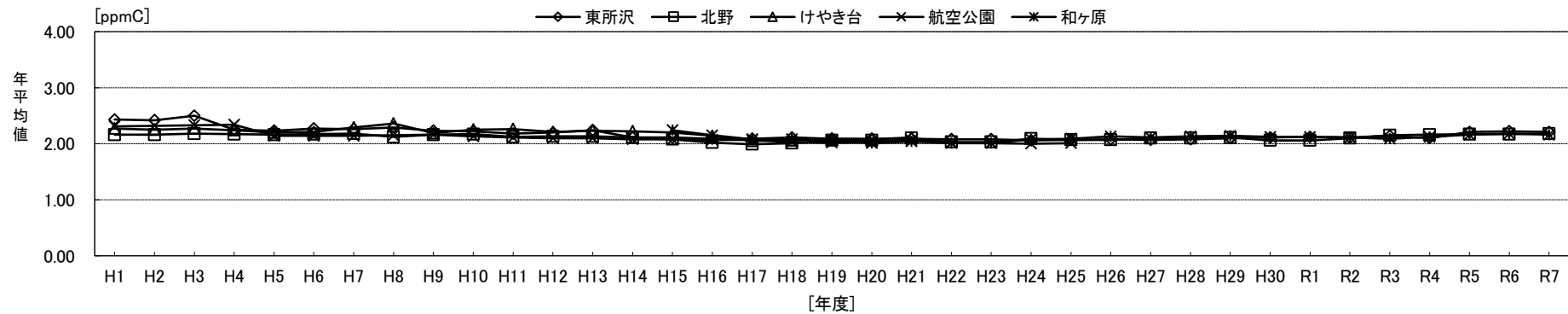
全炭化水素(THC)の経年変化
