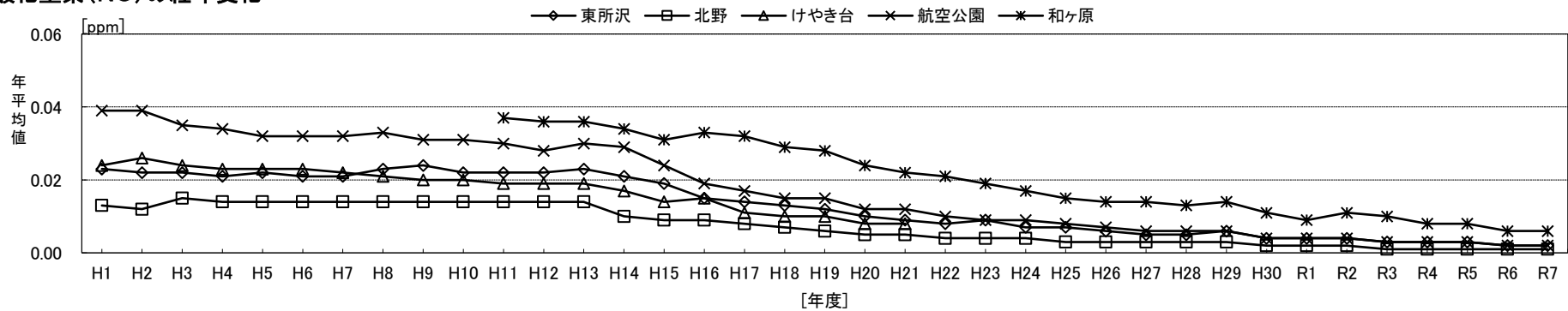
(b)一酸化窒素(NO)の月間値
