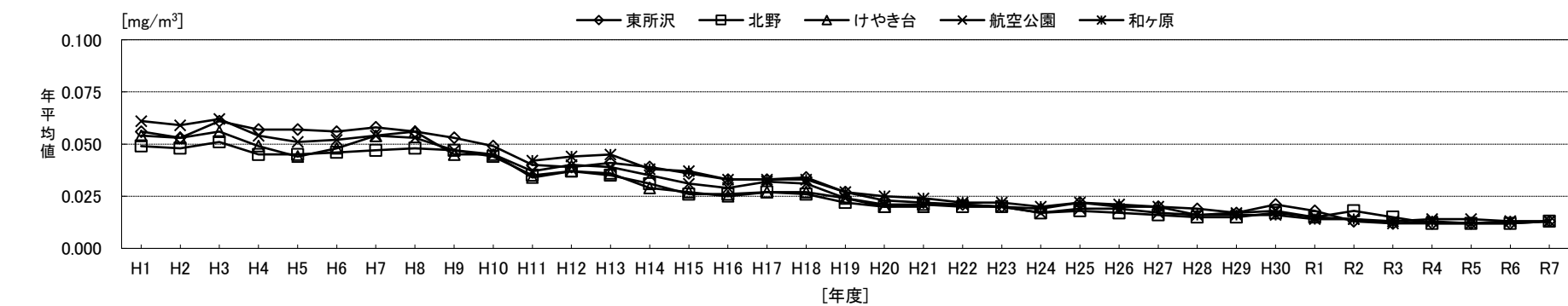
浮遊粒子状物質 (SPM)の経年変化
