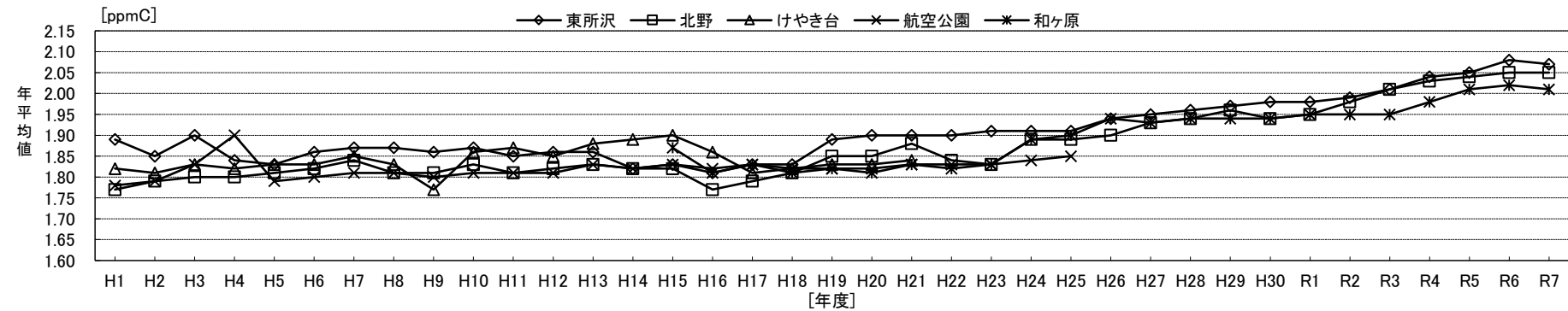
メタン(CH 4 )の経年変化
