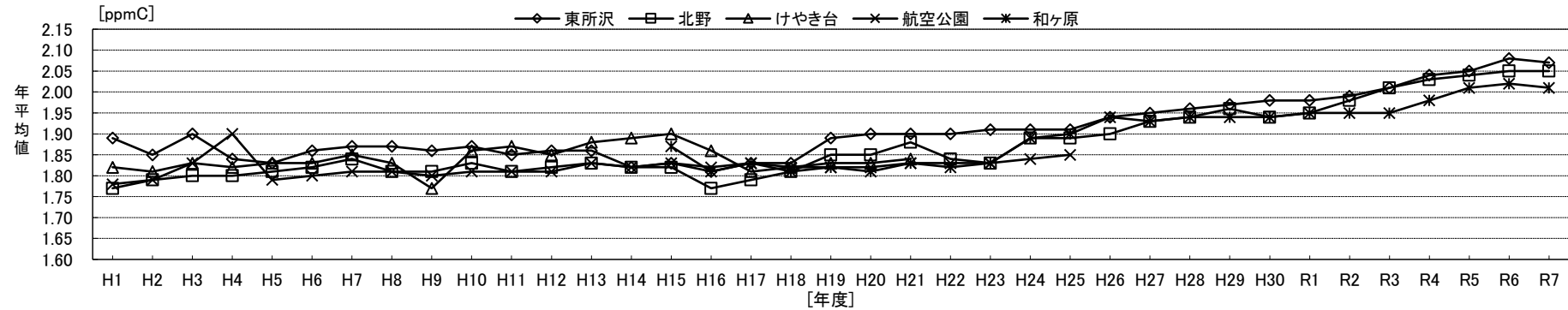
メタン(CH 4 )の経年変化
