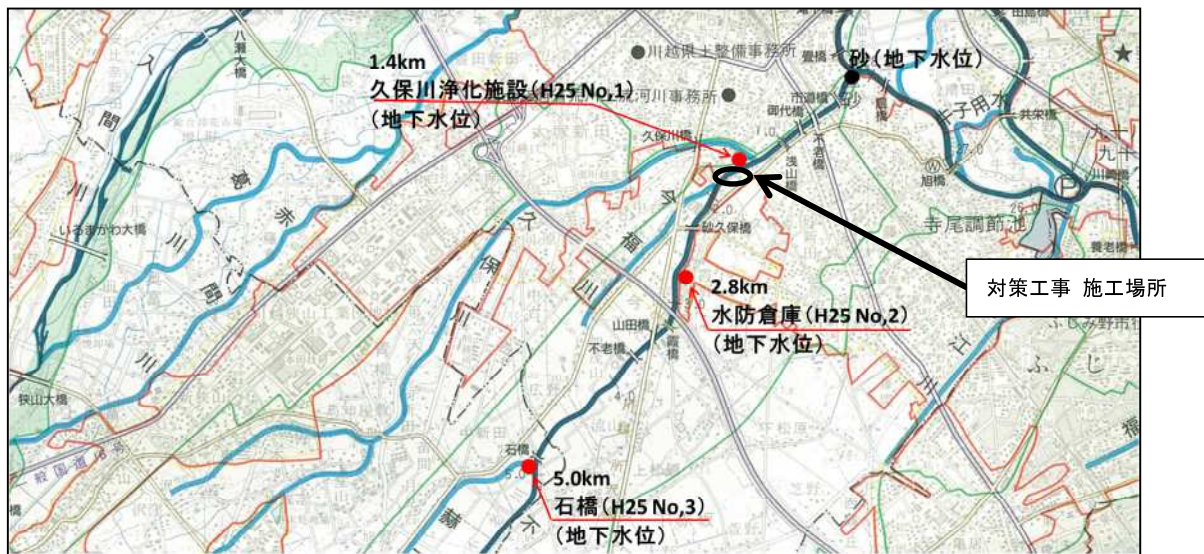
图 5.1 施工位置图
