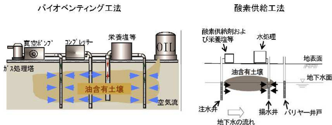
図 8-26 原位置バイオレメディエーションの概念図
