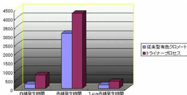
図 7-2 環境対応型技術の例 5)
