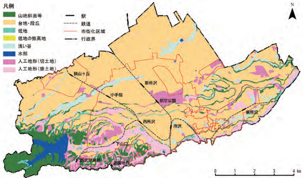
図 2-3 地形区分
