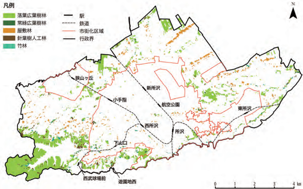
図 2-7 樹林の分布
