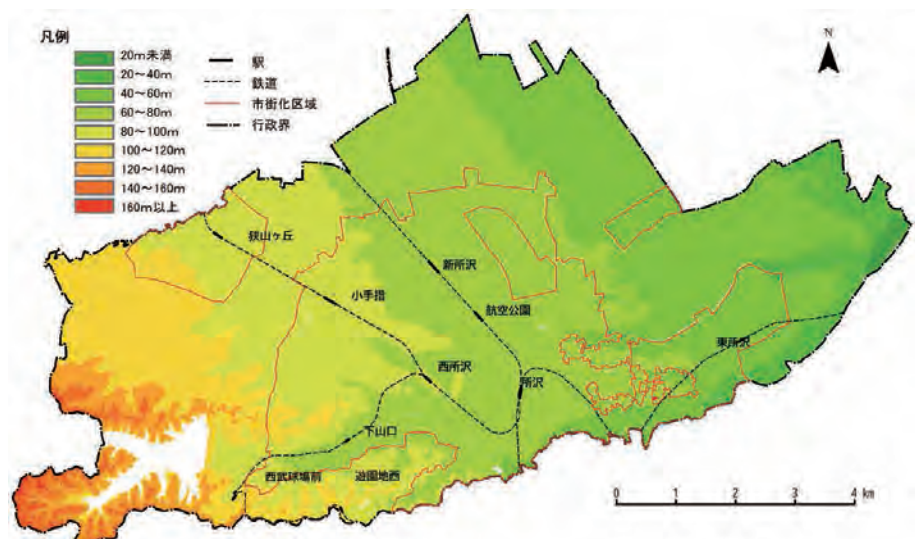
図2-2 標高
