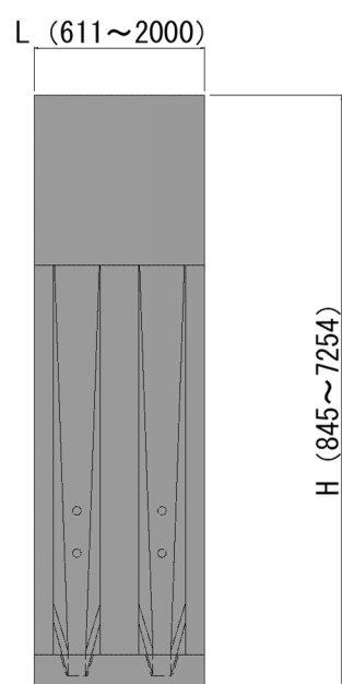
L 型擁壁
