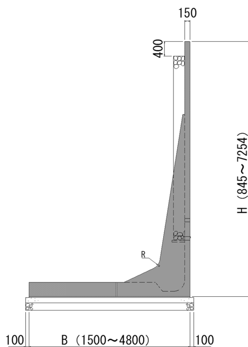
L 型擁壁
