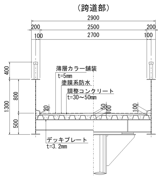
橋面補修工（断面図）
